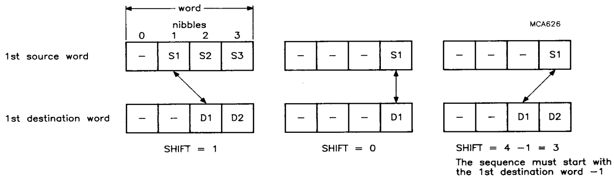
Fig.37 Shift example.
